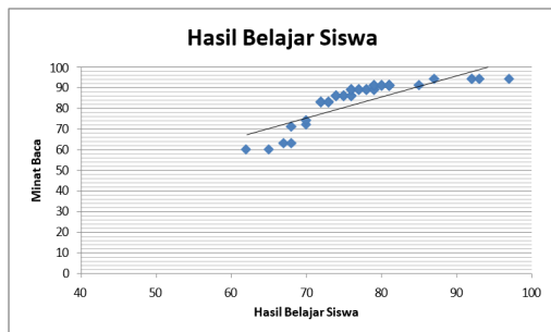
Gambar 1 Diagram Pancar Pengaruh Minat Baca (X) terhadap Hasil Belajar (Y)
