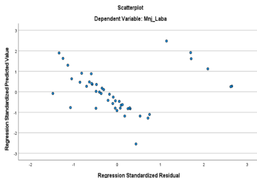
Gambar 4 Hasil Uji Heterokedastitas Sumber : Data Sekunder diolah menggunakan Alat Statistik
