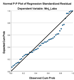
Gambar 2. Hasil Uji Normalitas setelah di outlier Sumber : Data sekunder diolah menggunakan Alat Statistik
