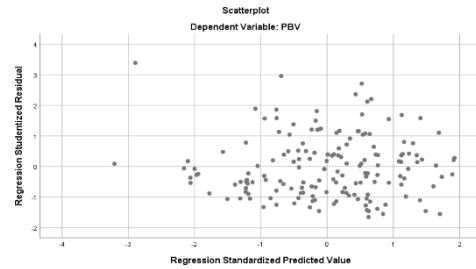
Gambar 1. Uji Heteroskedastisitas
