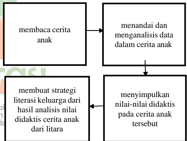
Diagram 1 Kerangka Berpikir
