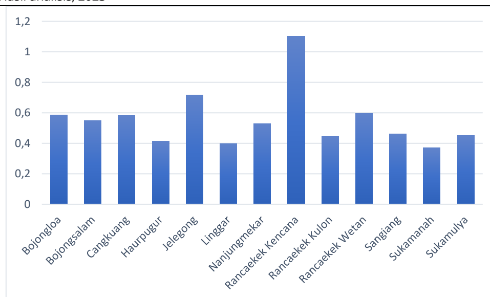
Gambar 2. Grafik Hasil penghitungan analisis nearest neighbor
